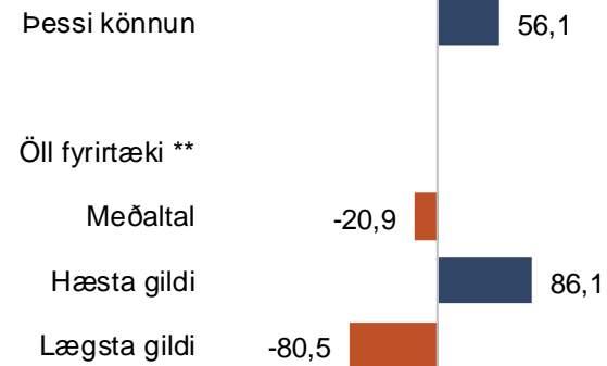
NPS (-100 til 100)
